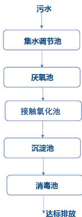
图 6 一体式废水处理设备处理流程图
