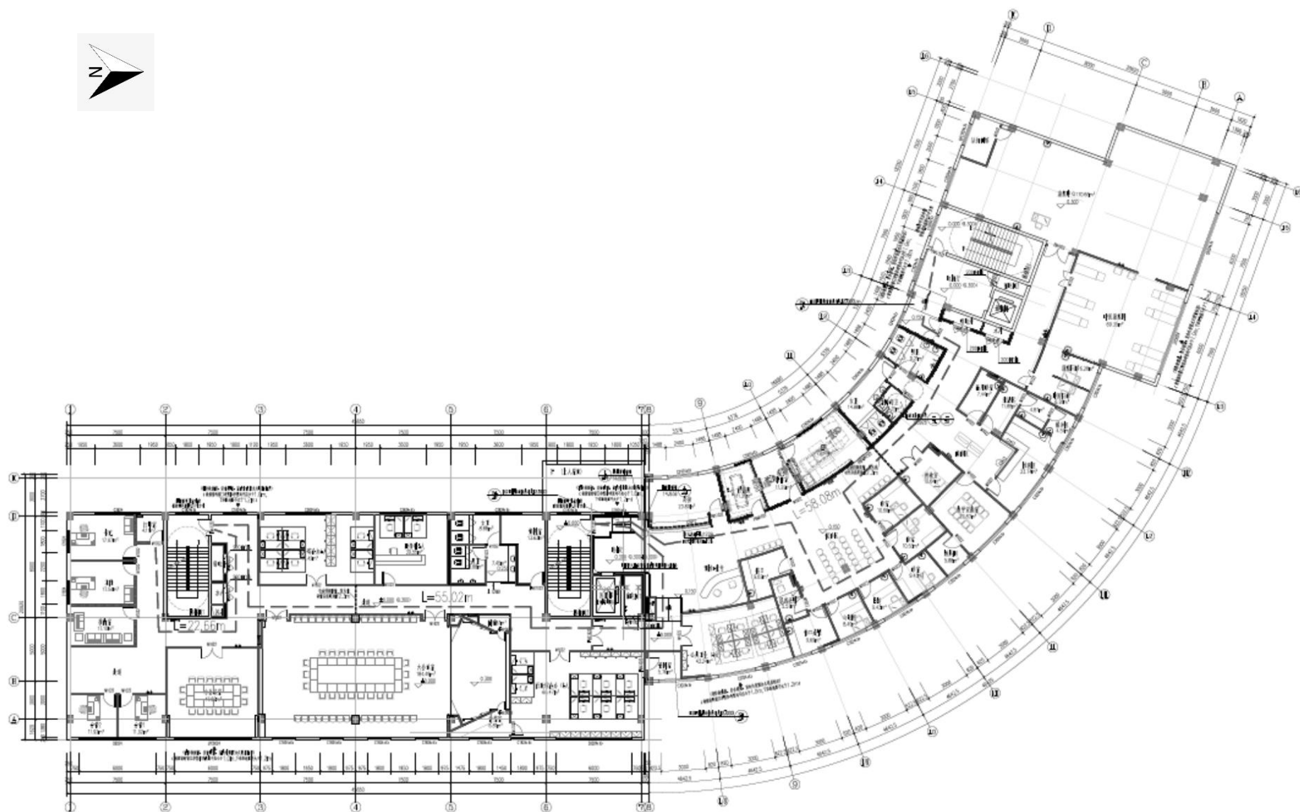
附图 5 本项目三层平面布置图
