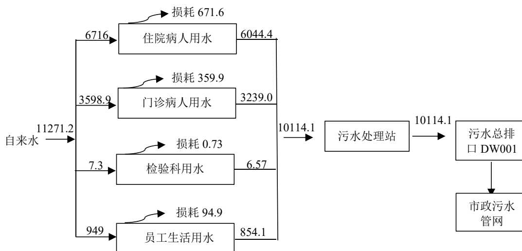
图2 本项目水平衡图 (单位: t/a)
